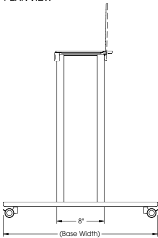
END ELEVATION
